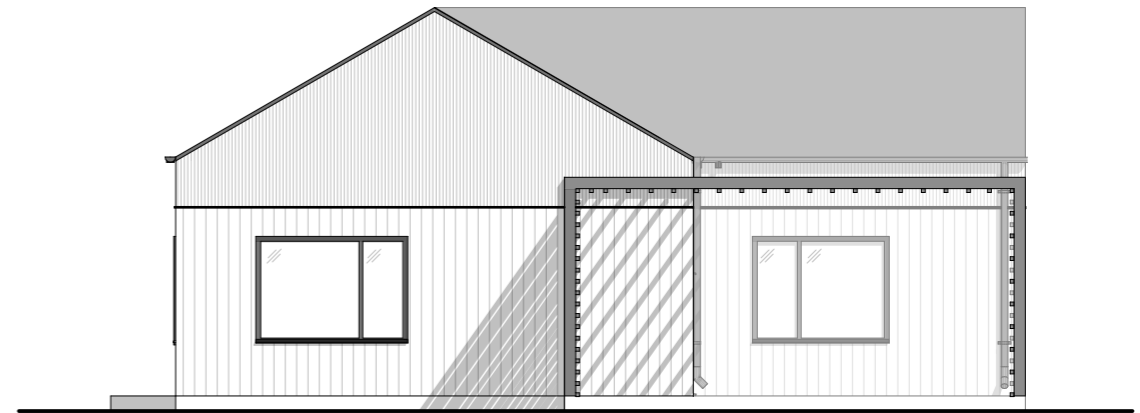
Fasad 2
